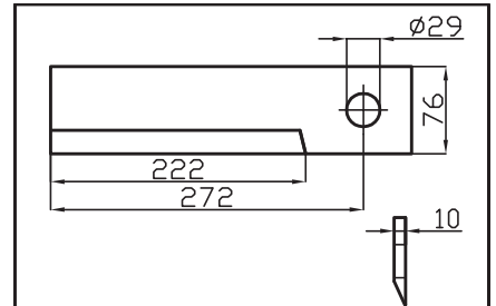
ON D2004 Izq.
